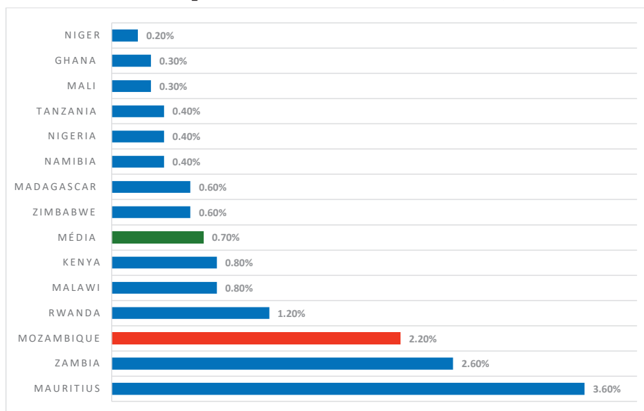
Gráfico 1: Total de perdas fiscais anuais (% do PIB)
